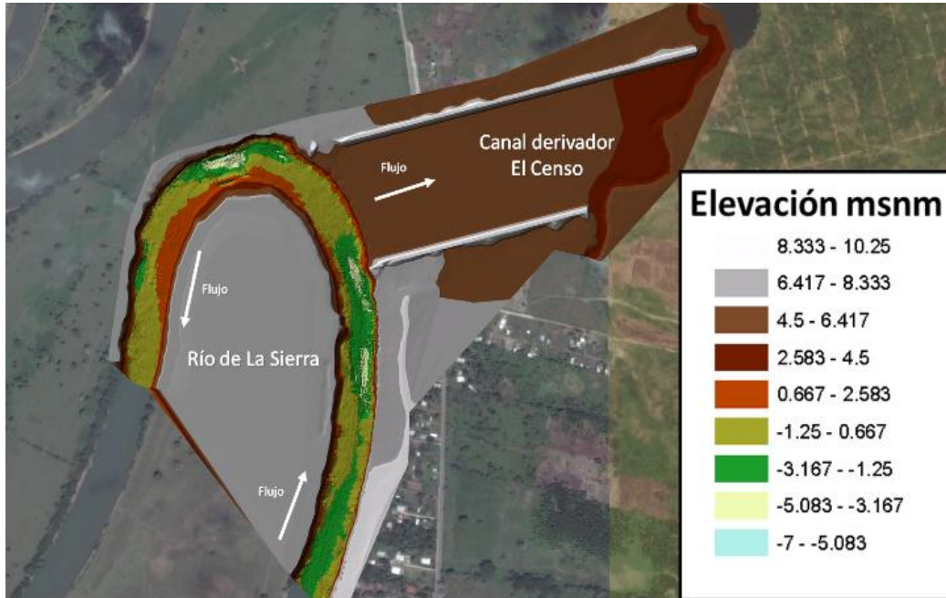
Figura 7. Batimetría del río La Sierra y canal derivador, El Censo.
