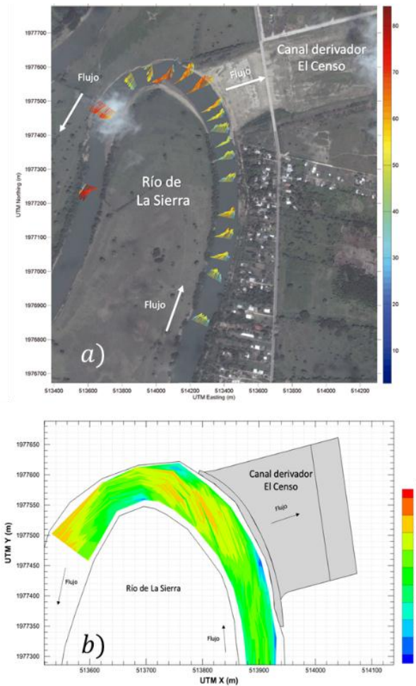
Figura 8. a) Vector de velocidad en planta del río La Sierra b) Magnitud de velocidad en planta del río La Sierra.
