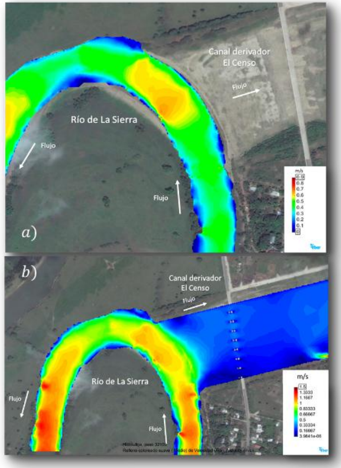
Figura 9. a) Modelo numérico del río La sierra en condición de gasto de Q = 109.0 \text{ m}^3\text{s}^{-1} .
